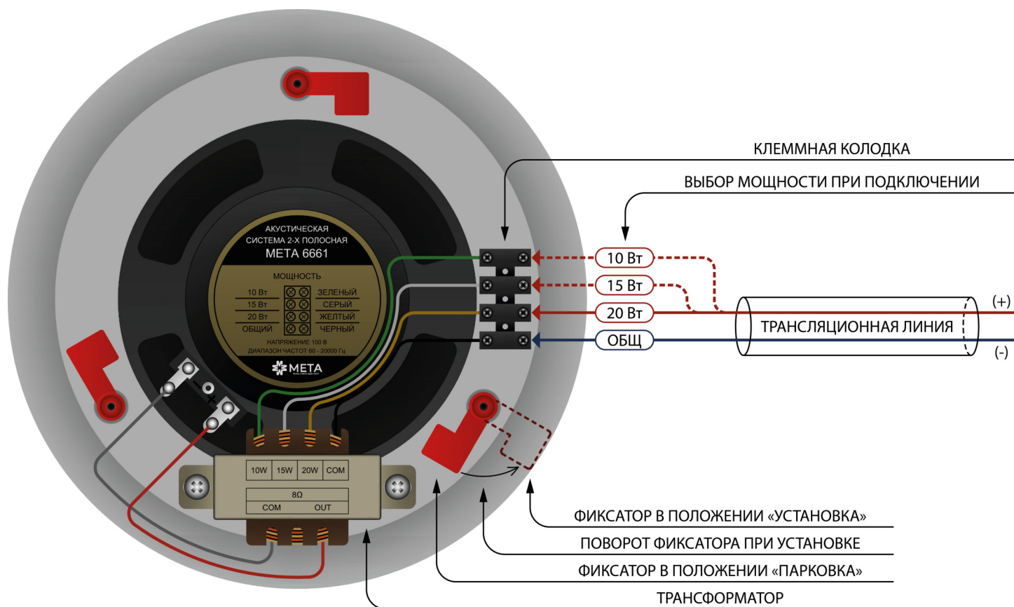
Рис. 3 Элементы крепления и коммутации БА
