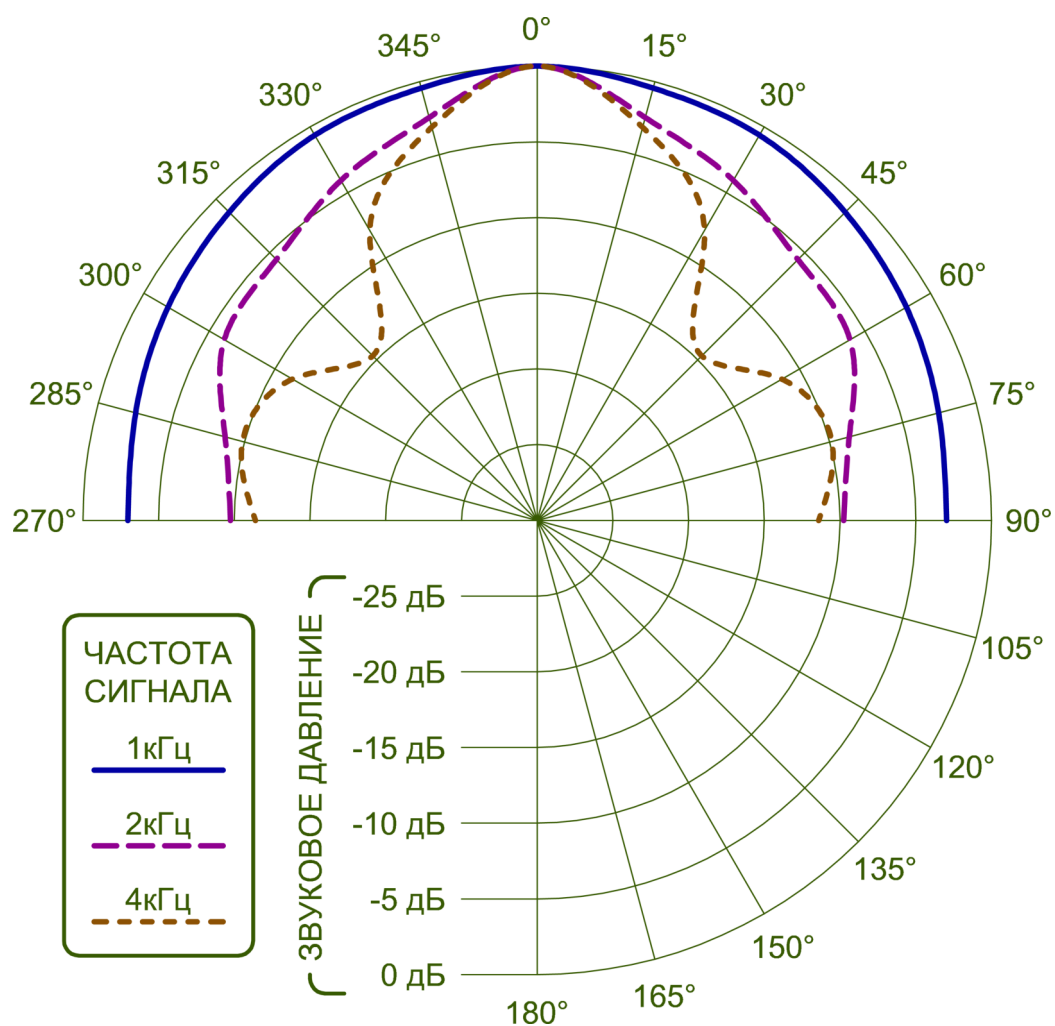
Рис.1 Характеристика направленности БА.
